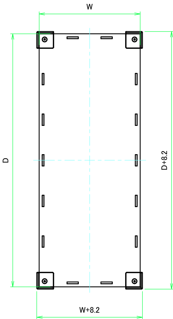
上カバー / Top cover
