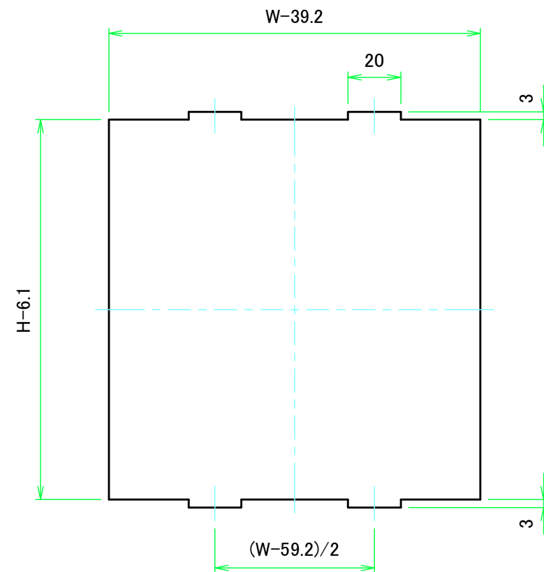
Wパネル1表面 / W Panel 1 Frontside
